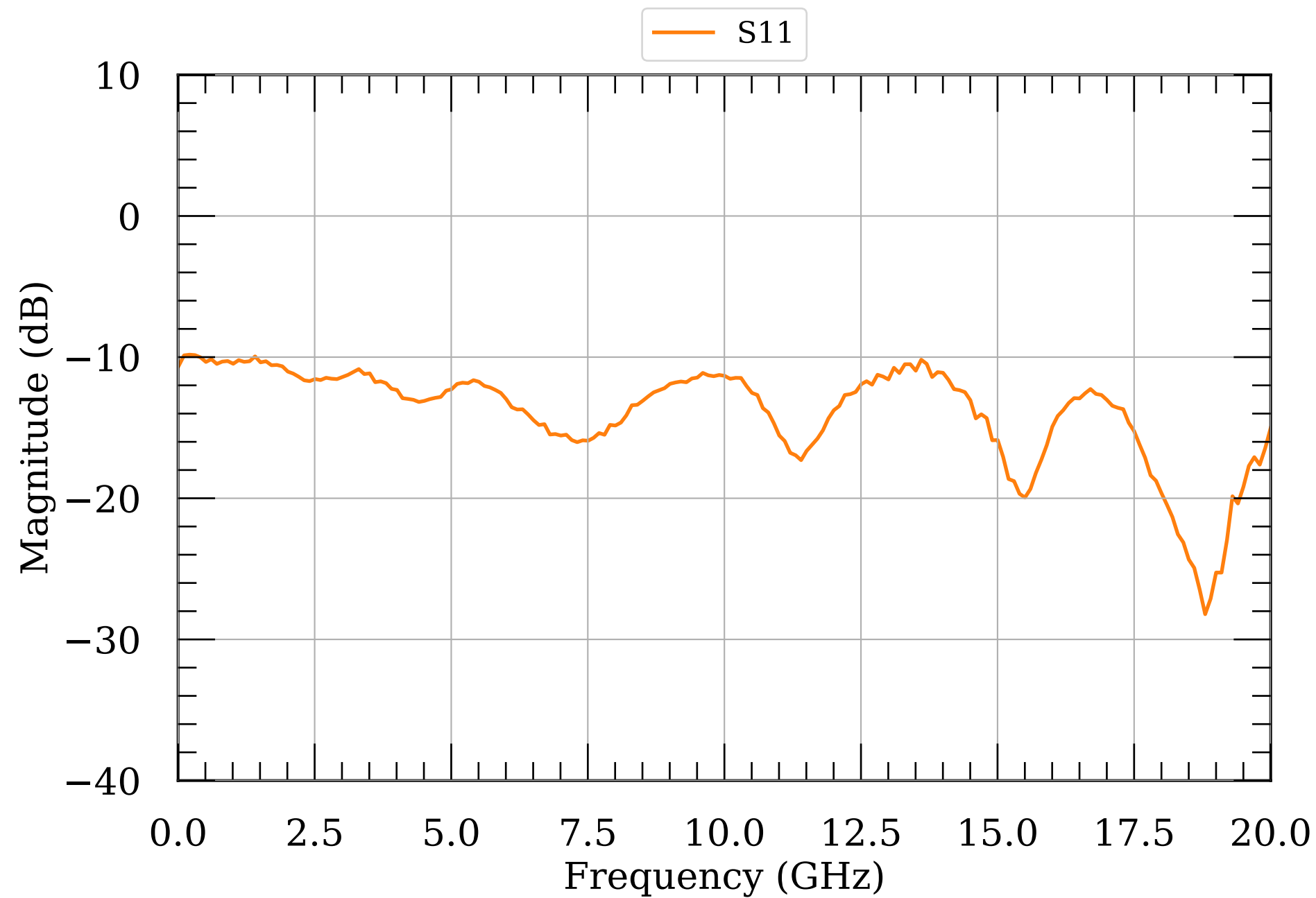
LNA S-params module048
